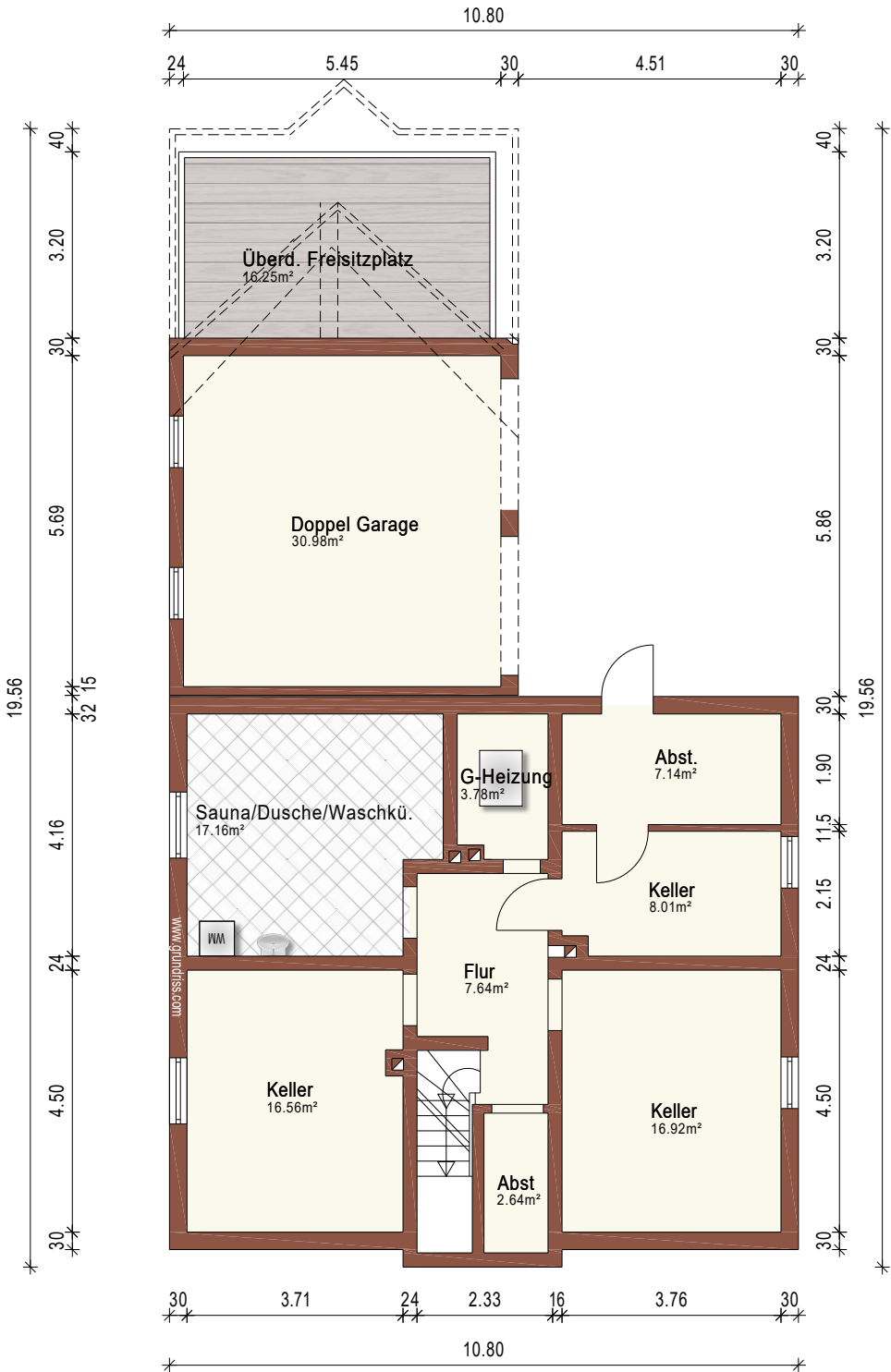
Kellergeschoss
